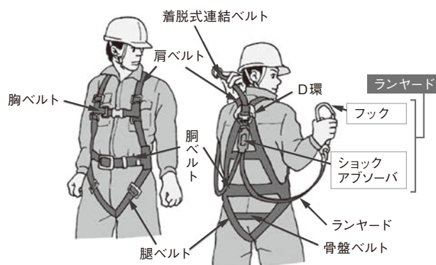
フルハーネス型墜落制止用器具の構成
